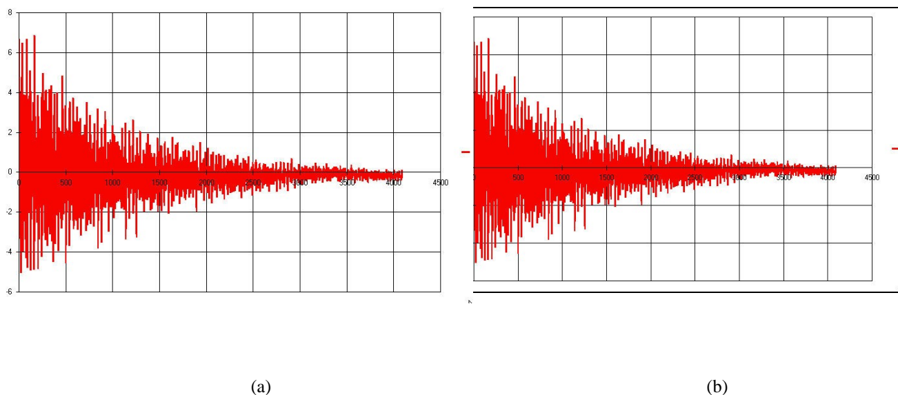
Fig. 3. Señal del acelerómetro (a) mosaico bueno, (b) mosaico defectuoso
